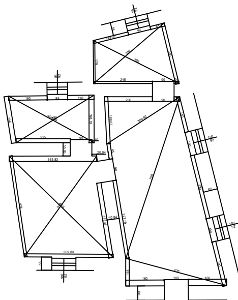
PIANTA APPARTAMENTO
